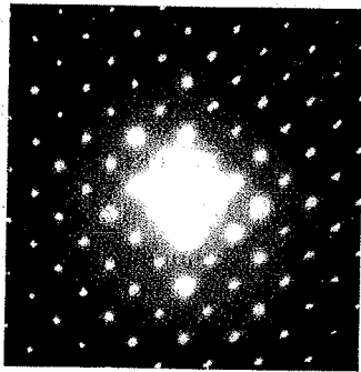
a. MoO 3 单晶的劳埃相
