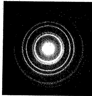
b. Au 多晶的德拜相
